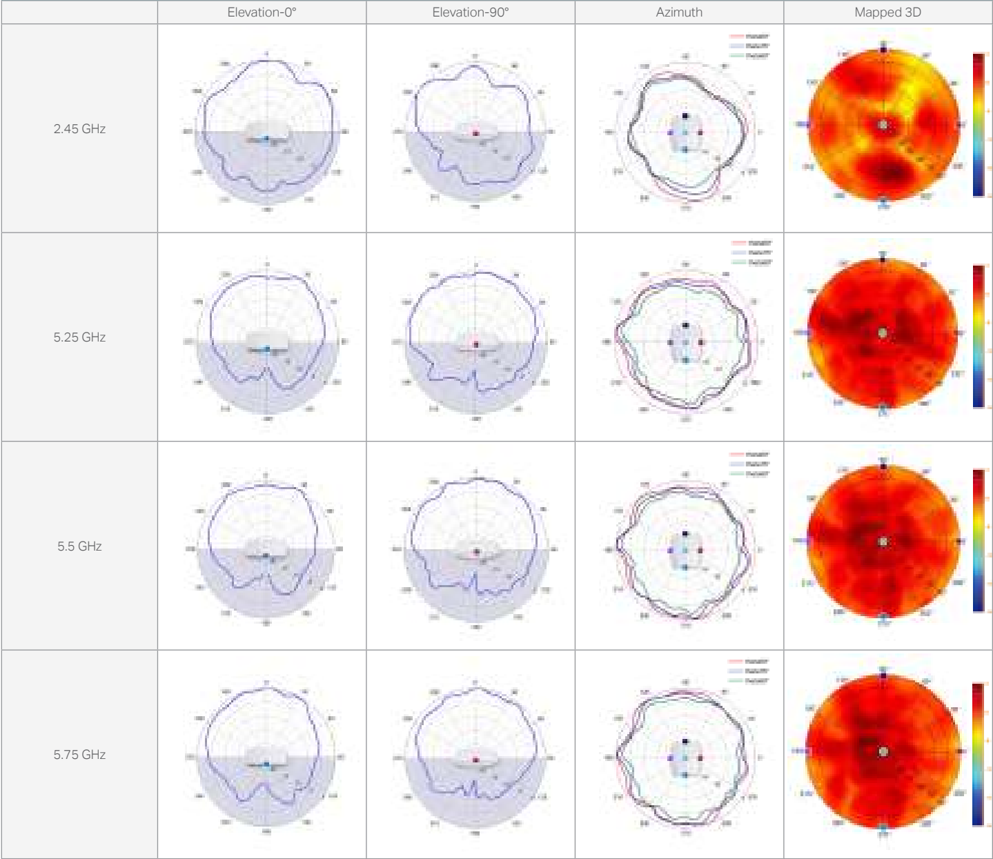
EAP265 HD
