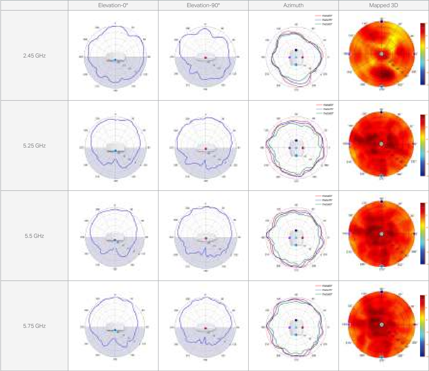
EAP245
