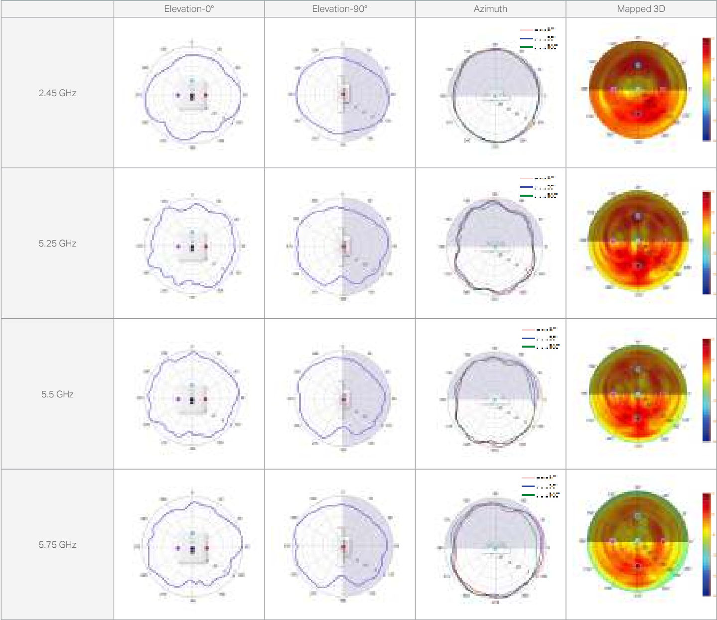
EAP230-Wall
