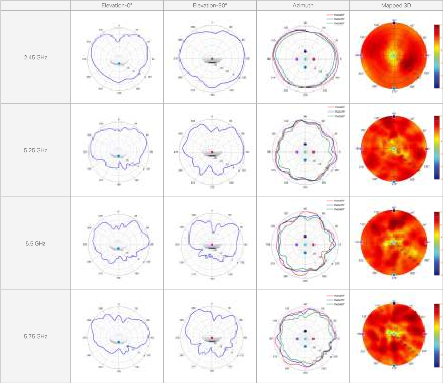
EAP620 HD
