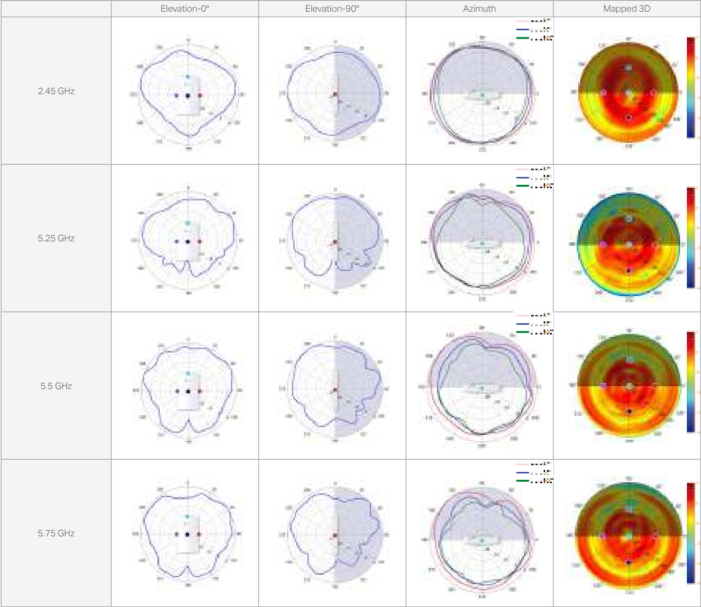
EAP235-Wall
