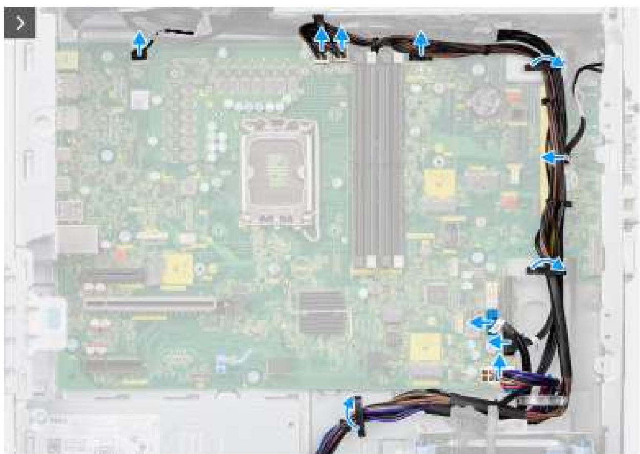
Figure 76. Retrait de la carte système
