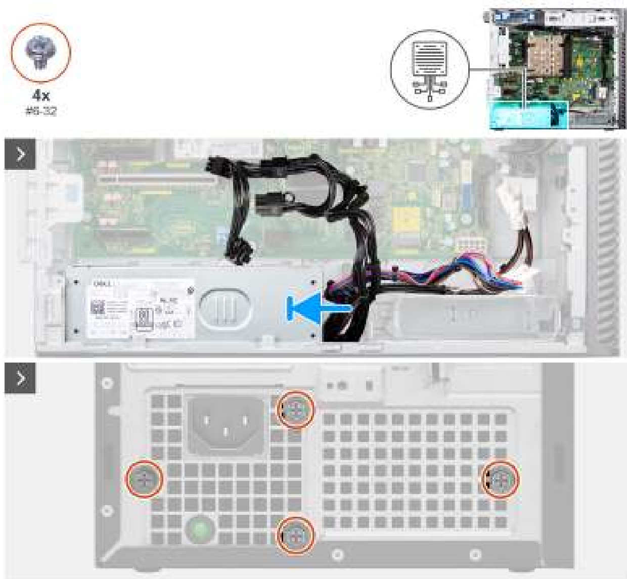
Figure 51. Installation du bloc d'alimentation de 1 000 W
