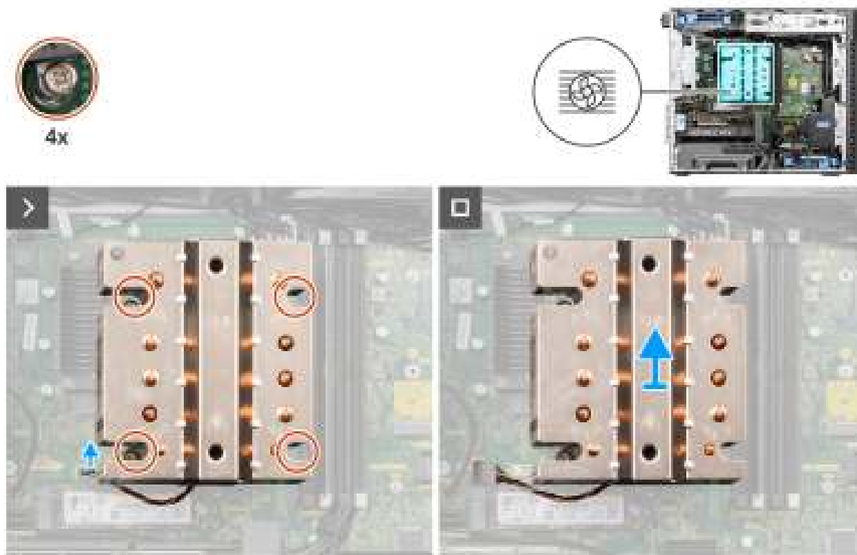
Figure 52. Retrait de l'assemblage du ventilateur et du dissipateur de chaleur 125 W du processeur
