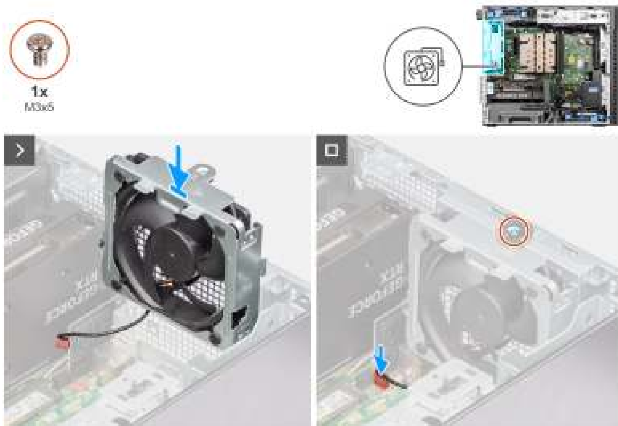
Figure 67. Installation du ventilateur arrière (bloc d'alimentation de 1 000 W)
