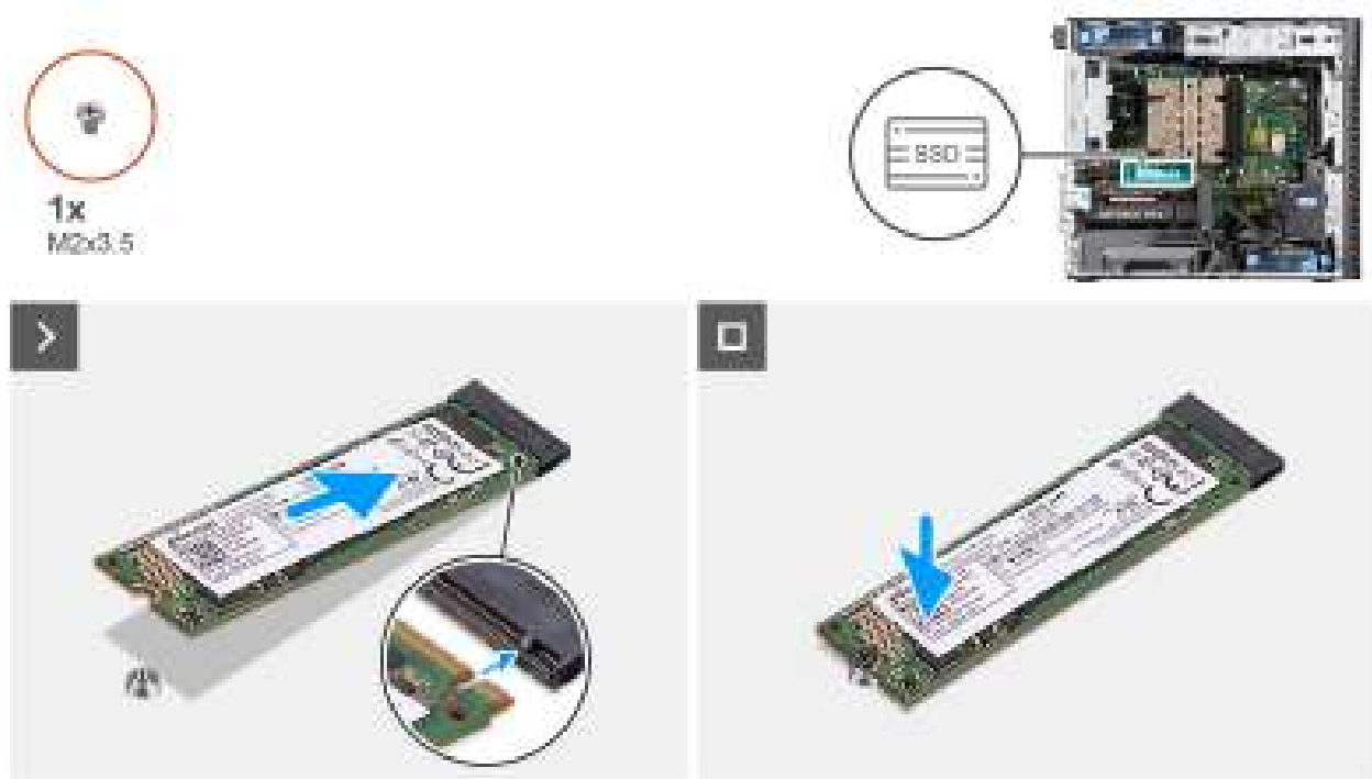
Figure 25. Installation du disque SSD M.2 2280 PCIe
