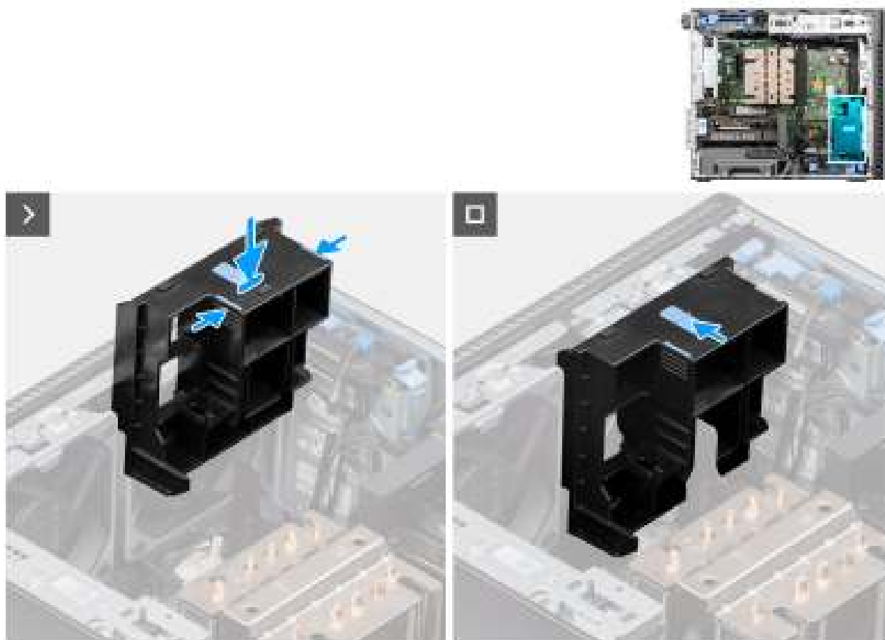
Figure 35. Installation du support d'extrémité du processeur graphique
