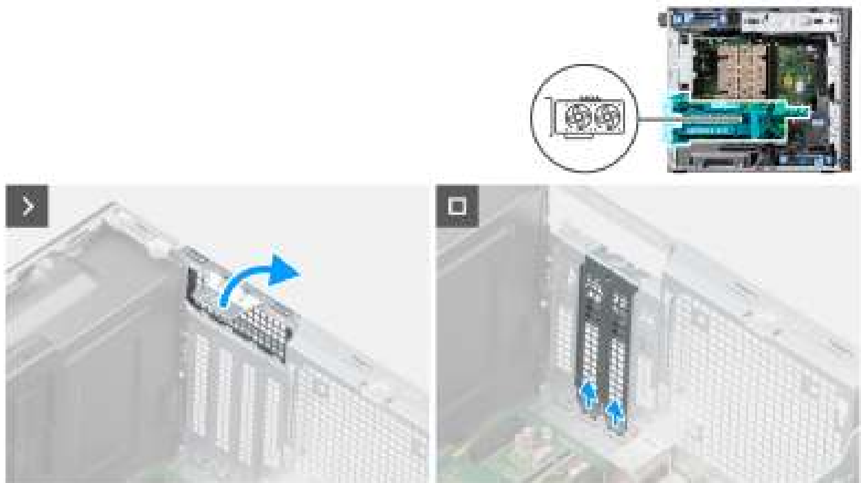
Figure 43. Installation du processeur graphique alimenté
