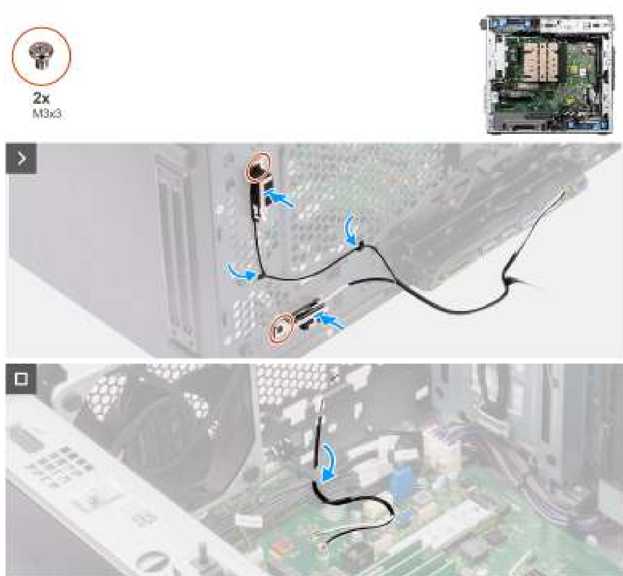
Figure 29. Installation de l'antenne interne WLAN
