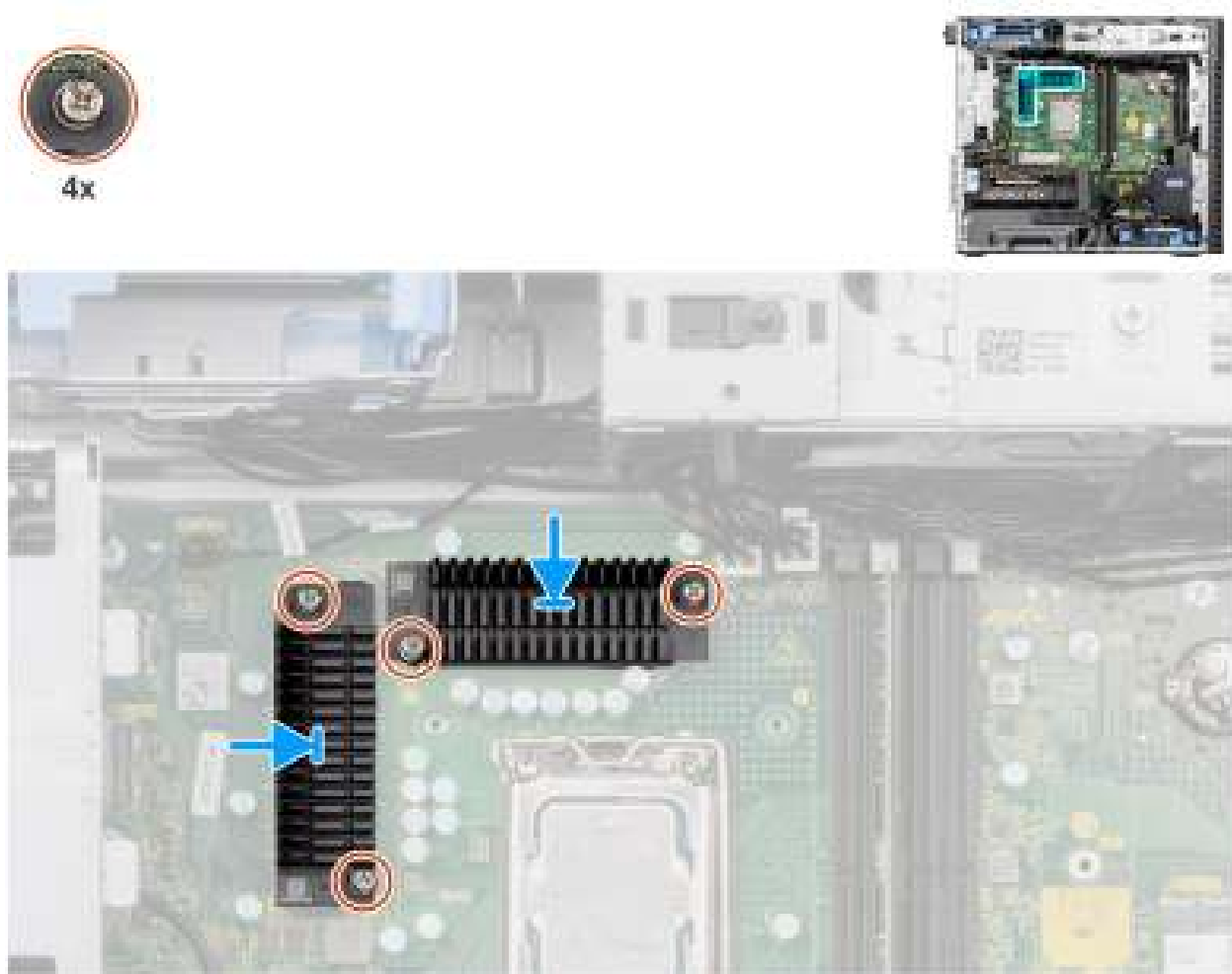
Figure 59. Installation du dissipateur de chaleur du régulateur de tension
