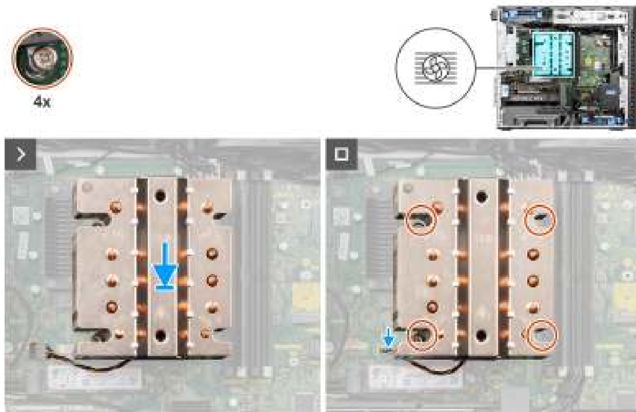
Figure 53. Installation de l'assemblage du ventilateur et du dissipateur de chaleur 125 W du processeur
