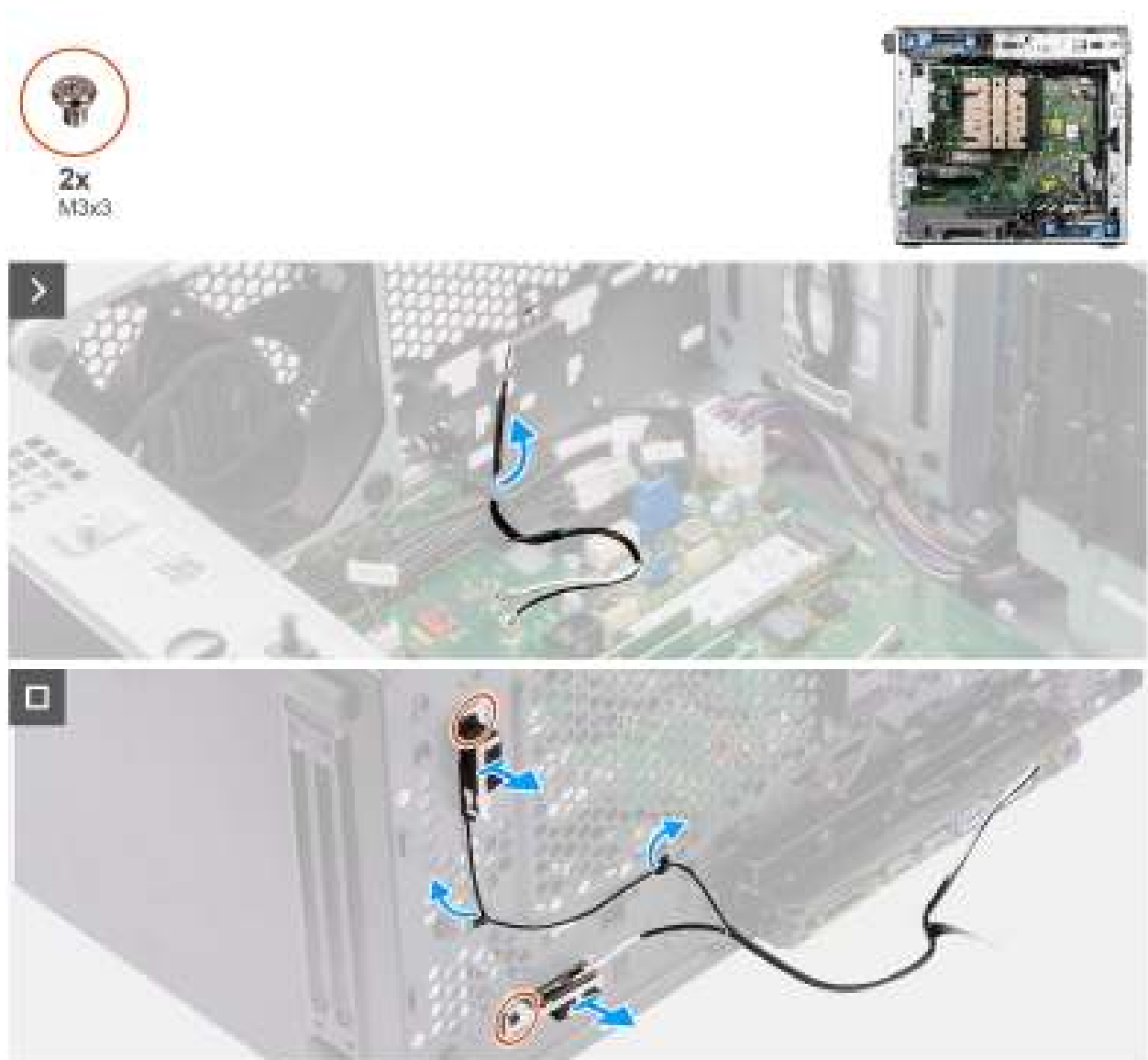
Figure 28. Retrait de l'antenne interne WLAN
