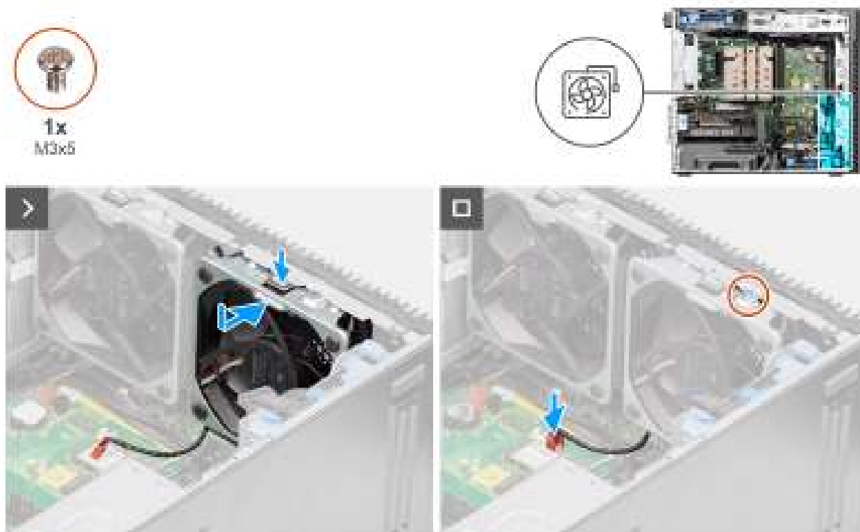
Figure 62. Ventilateur avant 1
