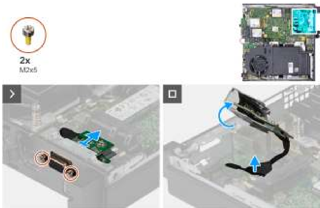
Figure 35. Retrait du module d'E/S en option (VGA ou série)
