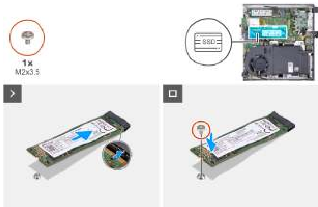
Figure 22. Installation du disque SSD M.2 2280 dans le logement 0
