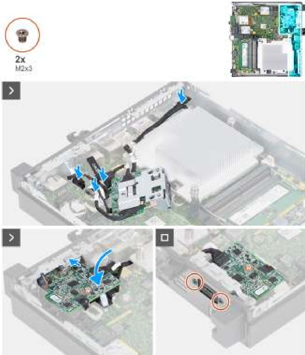
Figure 39. Installation du module USB-C en option
