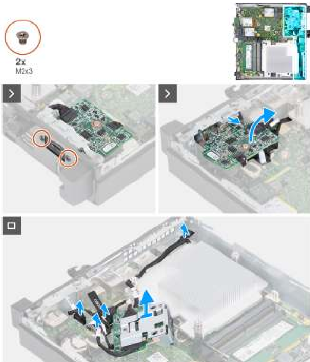
Figure 38. Retrait du module USB-C en option
