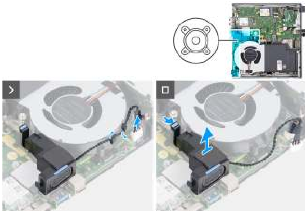
Afbeelding 17. De luidspreker verwijderen
