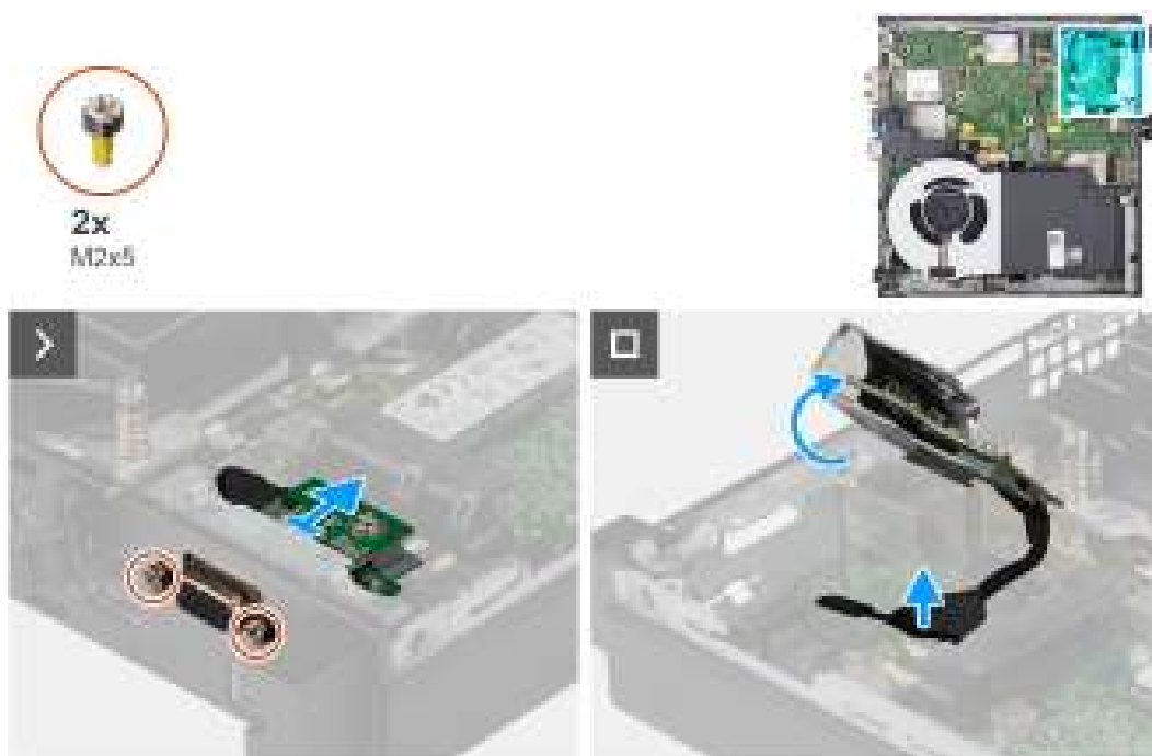
Afbeelding 35. De optionele I/O-module verwijderen (VGA of serieel)
