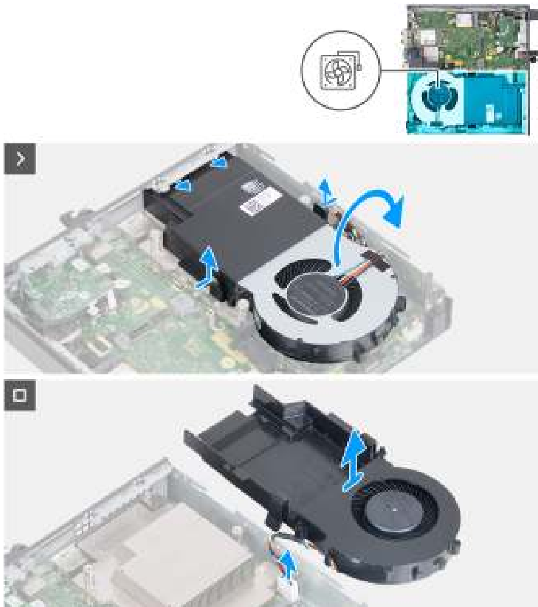
Afbeelding 30. De ventilator verwijderen
