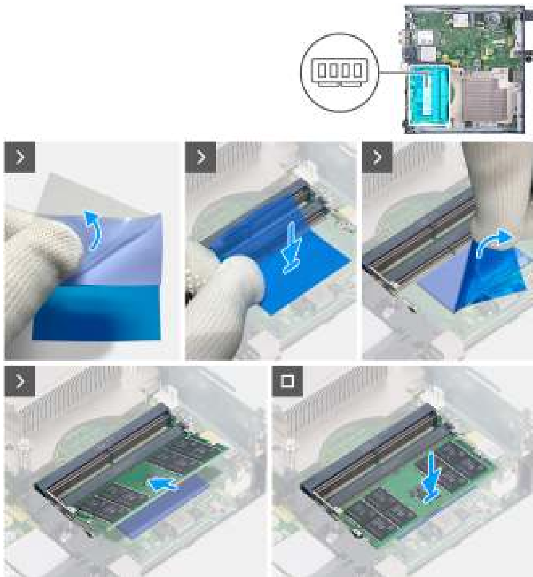
Afbeelding 33. De geheugenmodule plaatsen
