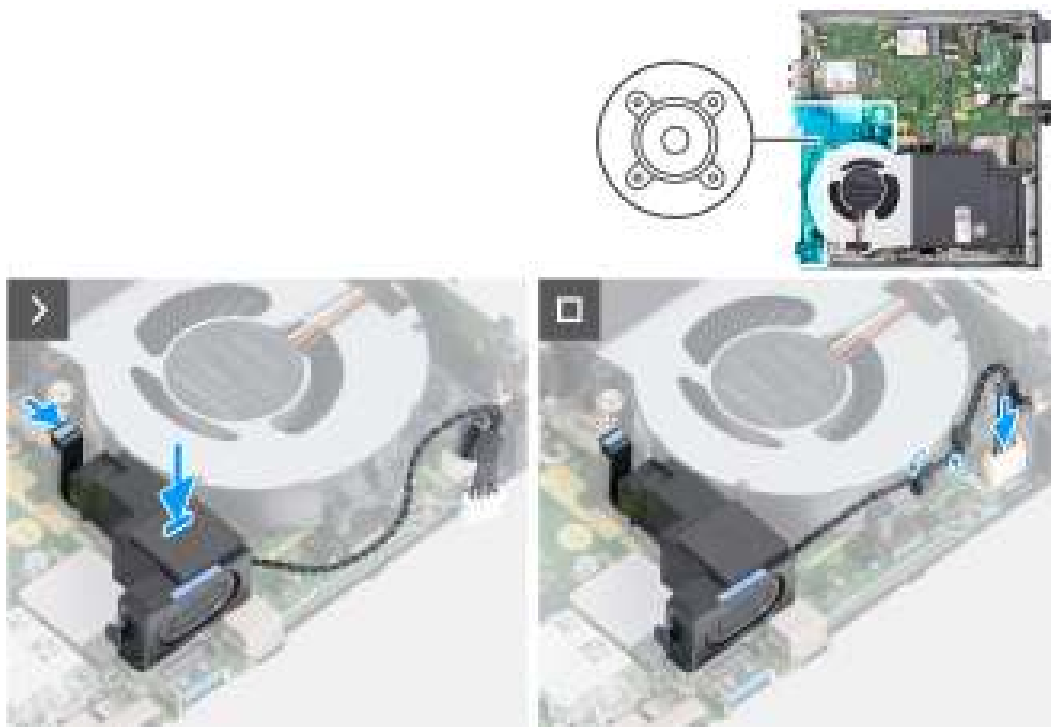
Afbeelding 18. De luidspreker plaatsen
