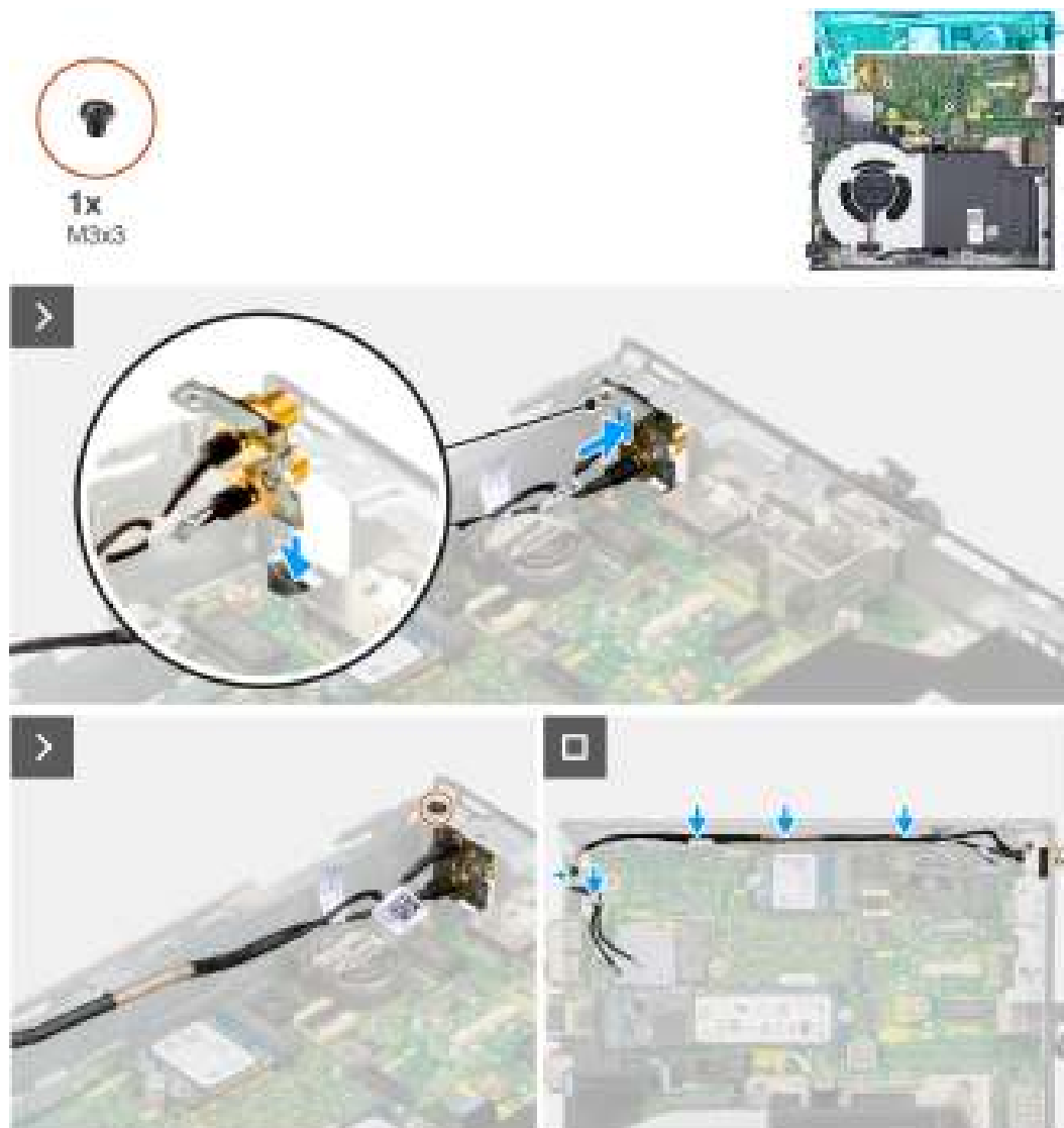
Afbeelding 55. SMA-antenne installeren (locatie 3)
