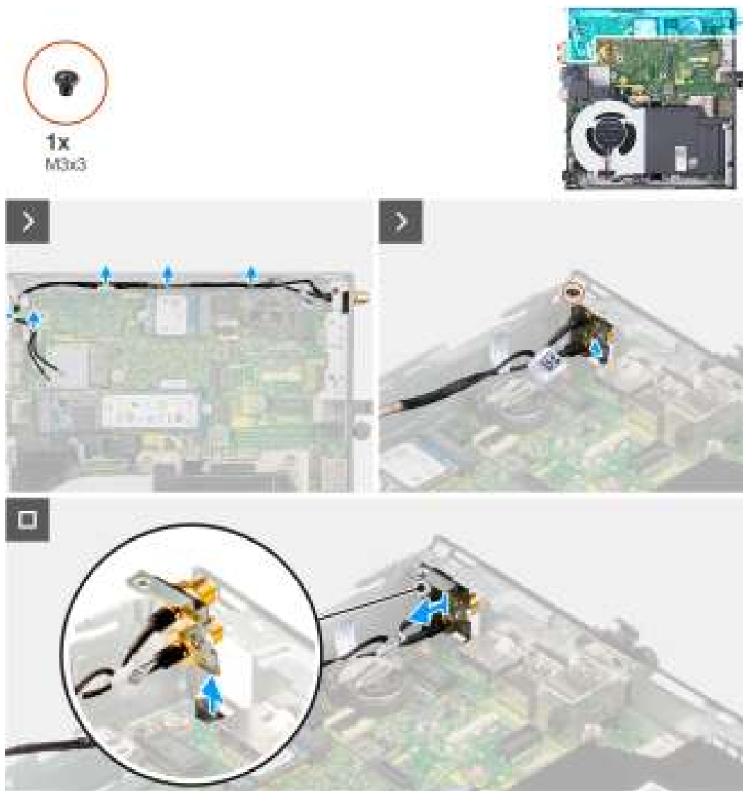
Afbeelding 54. De SMA-antenne verwijderen
