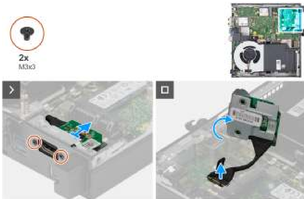
Afbeelding 34. De optionele I/O-module verwijderen (HDMI, DP of PS2)
