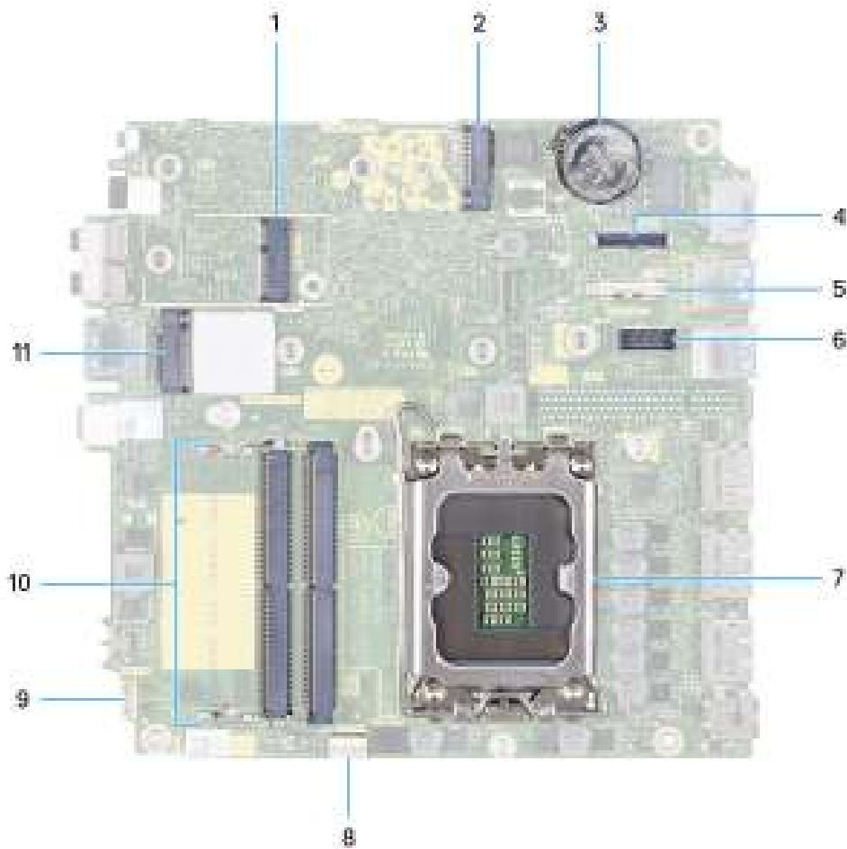
Afbeelding 44. Systeemkaartconnectoren
