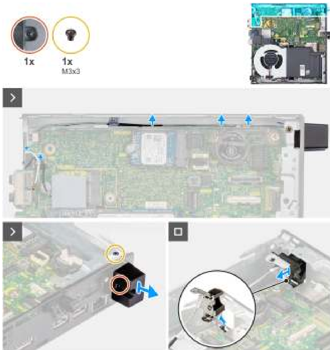
Afbeelding 50. De antennemodule (witte kabel) verwijderen
