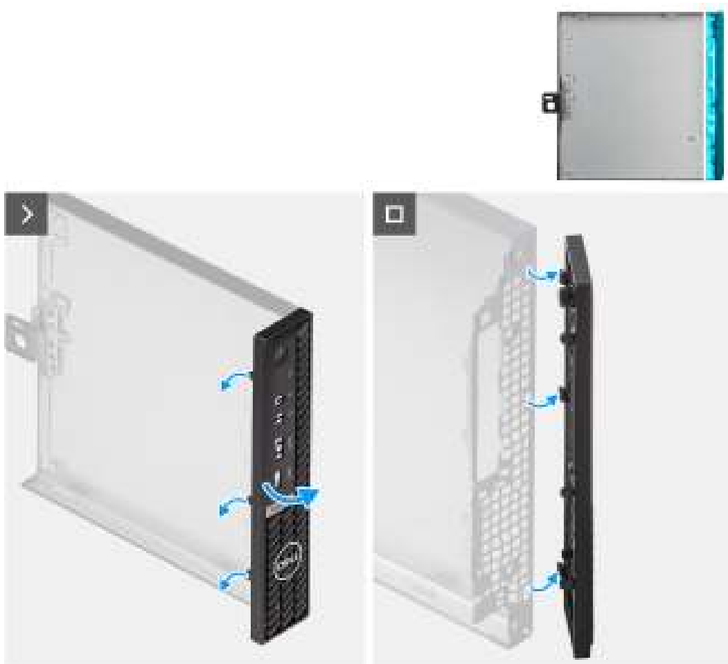
Afbeelding 15. Het montagekader aan de voorkant verwijderen
