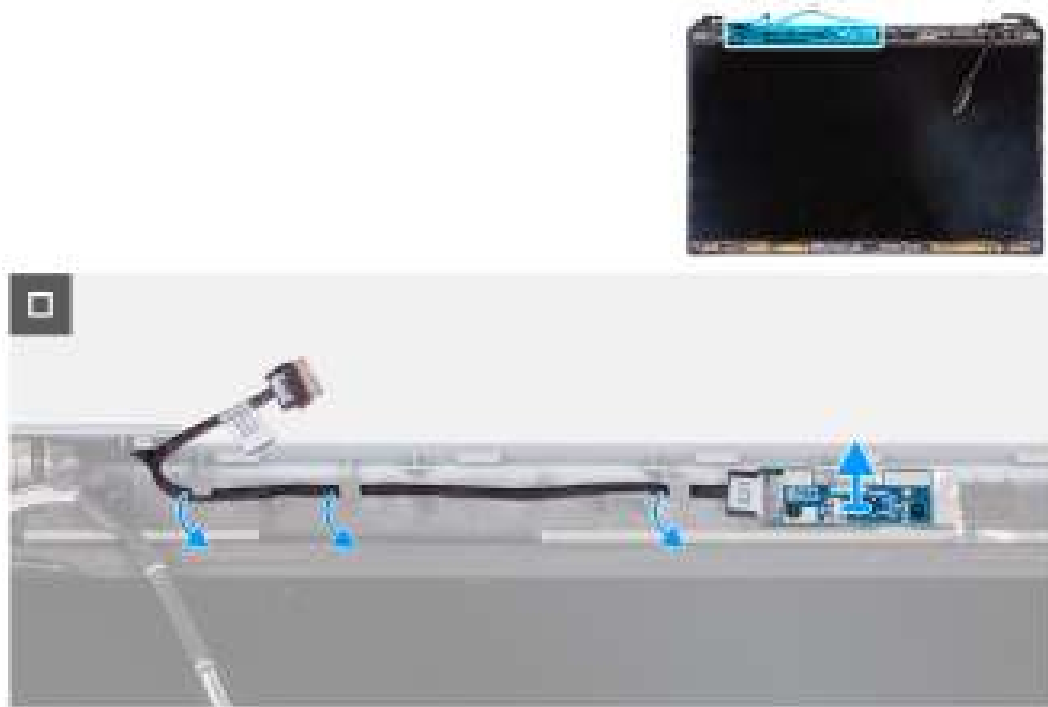
Afbeelding 92. De sensorkaart verwijderen
