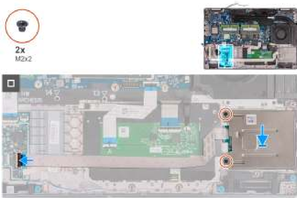
Afbeelding 97. De smartcardlezer plaatsen
