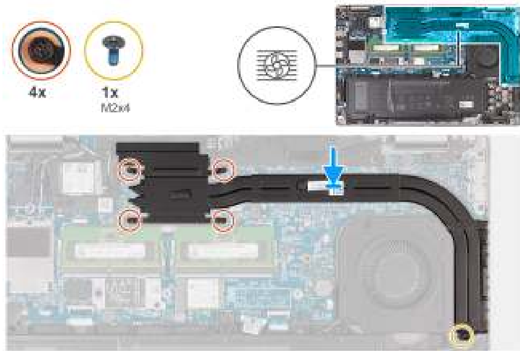
Afbeelding 51. De koelplaat installeren (geïntegreerde GPU)
