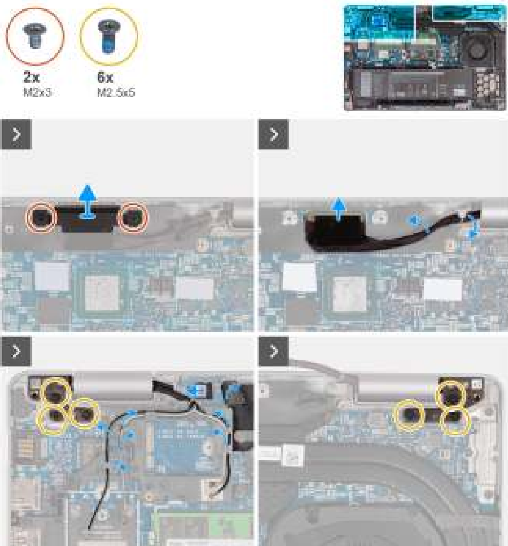
Afbeelding 69. De beeldschermeenheid verwijderen
