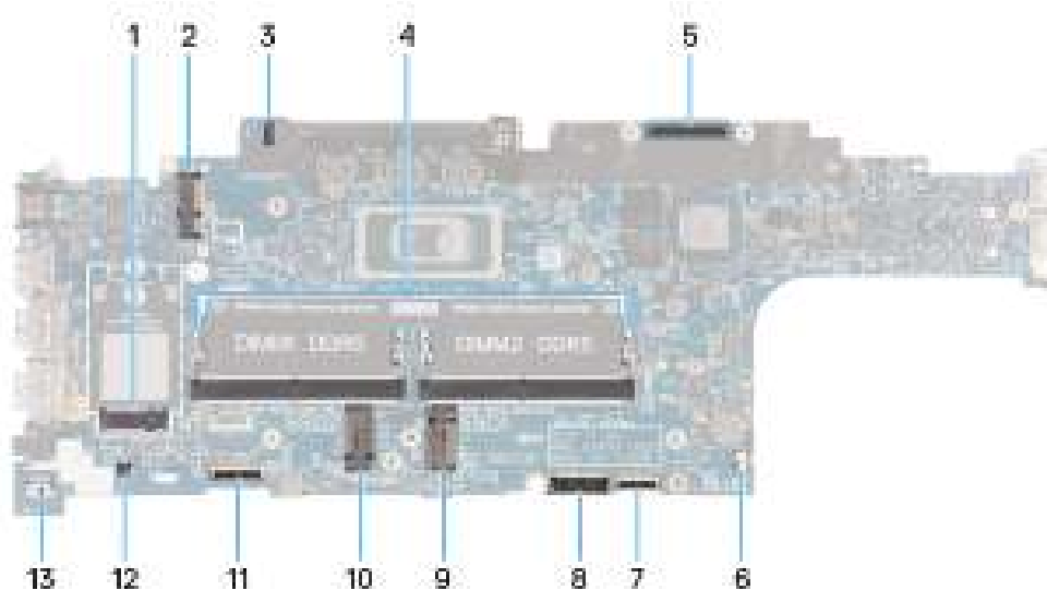
Afbeelding 57. Systeemkaartconnectoren
