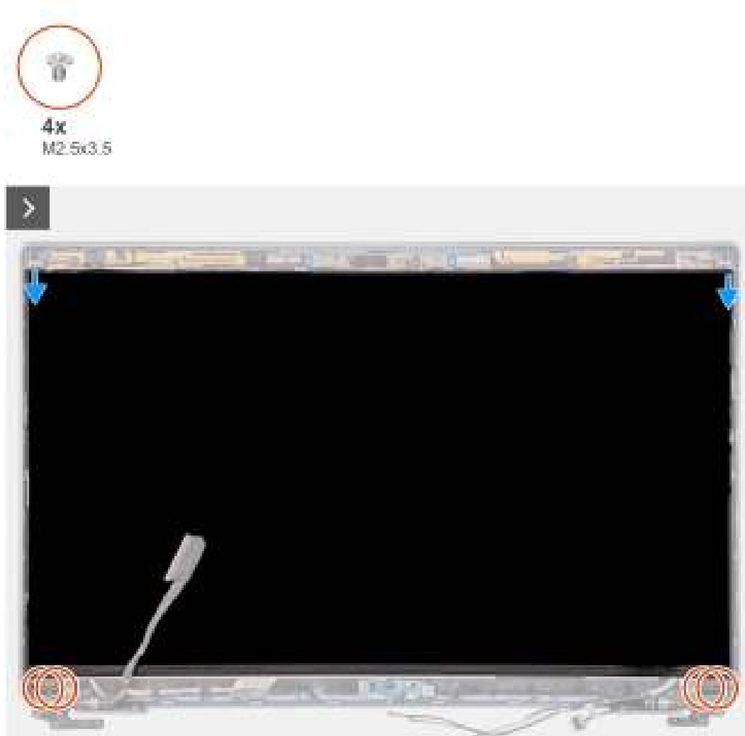
Afbeelding 76. Het beeldschermpaneel verwijderen
