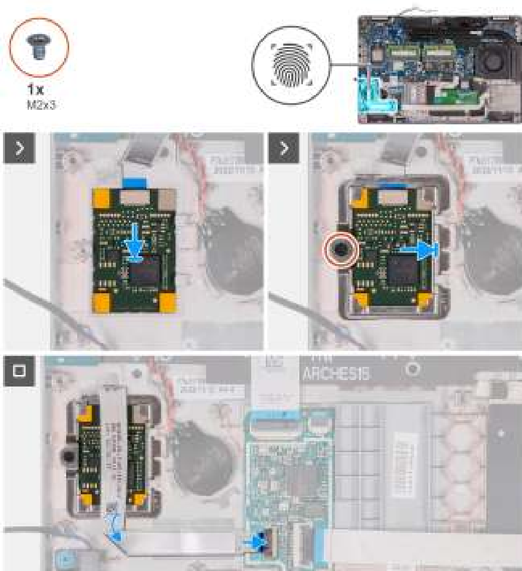
Afbeelding 95. De vingerafdrukkelezer plaatsen
