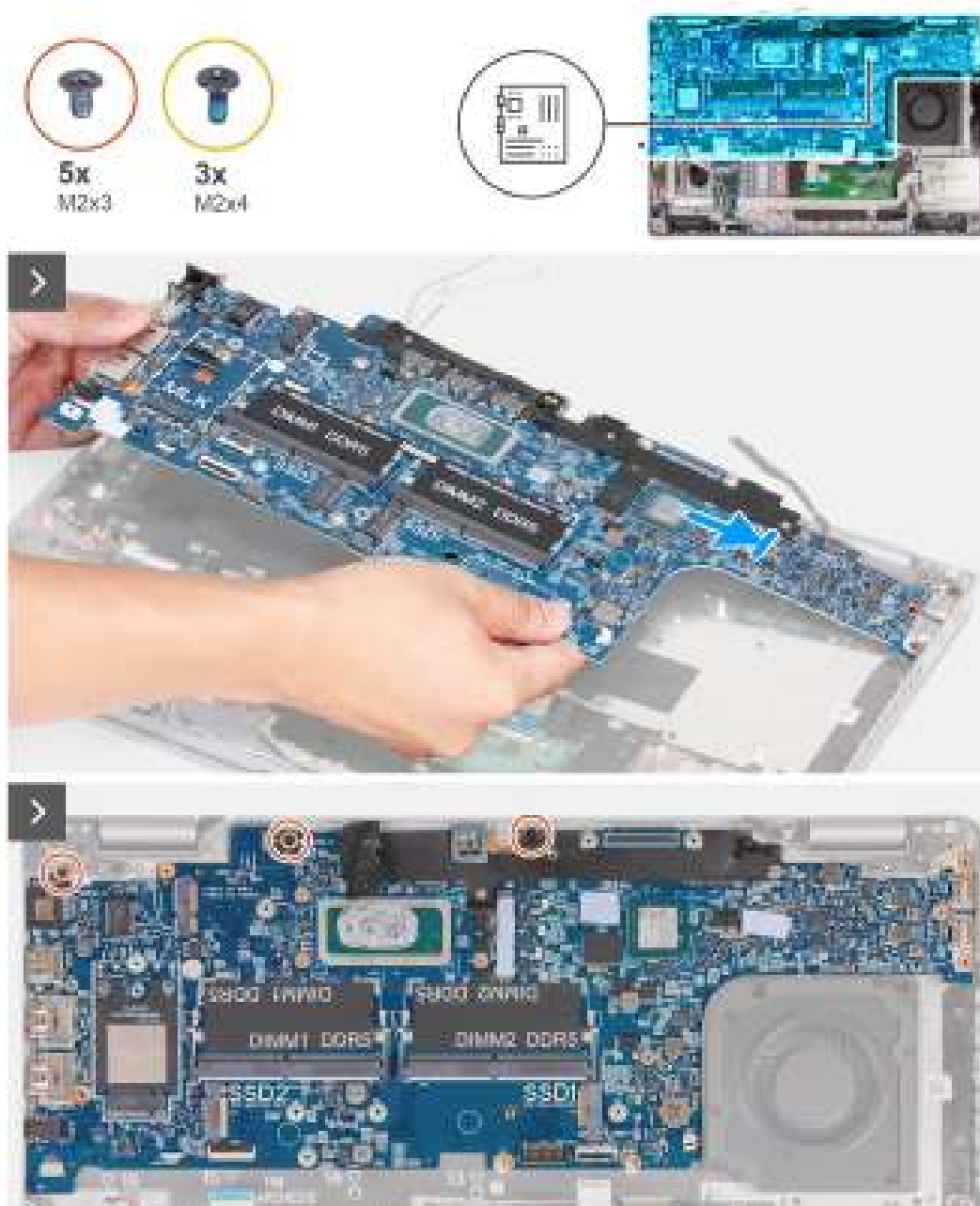
Afbeelding 58. De systeemkaart installeren
