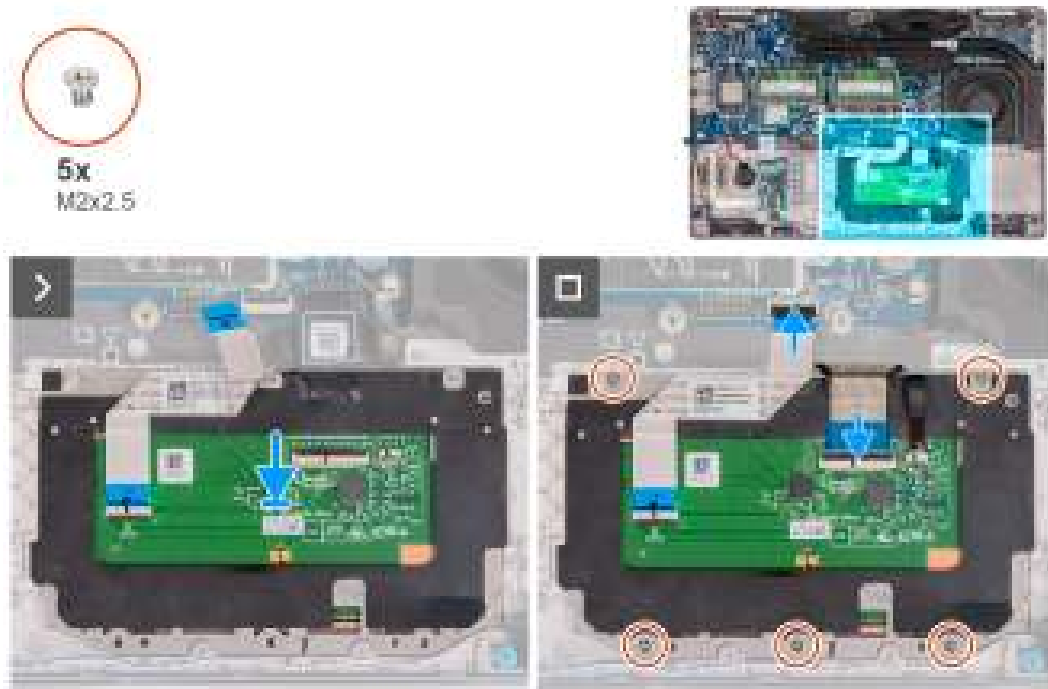
Afbeelding 42. De touchpad installeren
