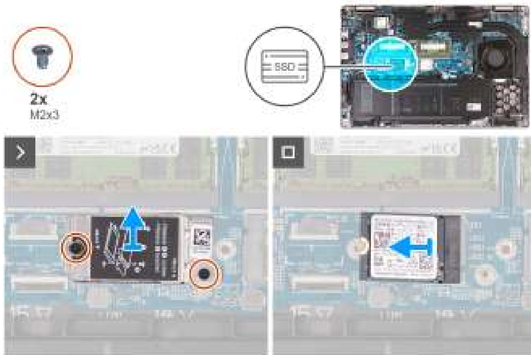
Afbeelding 32. De M.2 2230 SSD in slot 2 installeren
