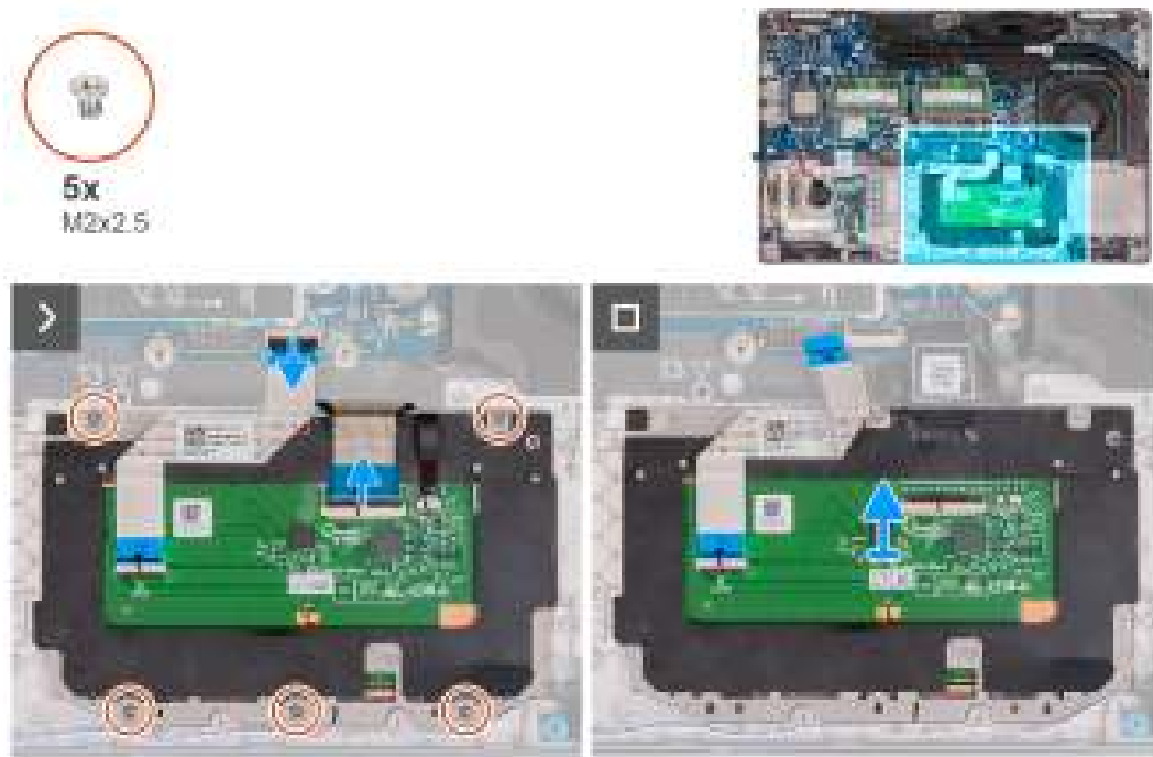
Afbeelding 41. De touchpad verwijderen
