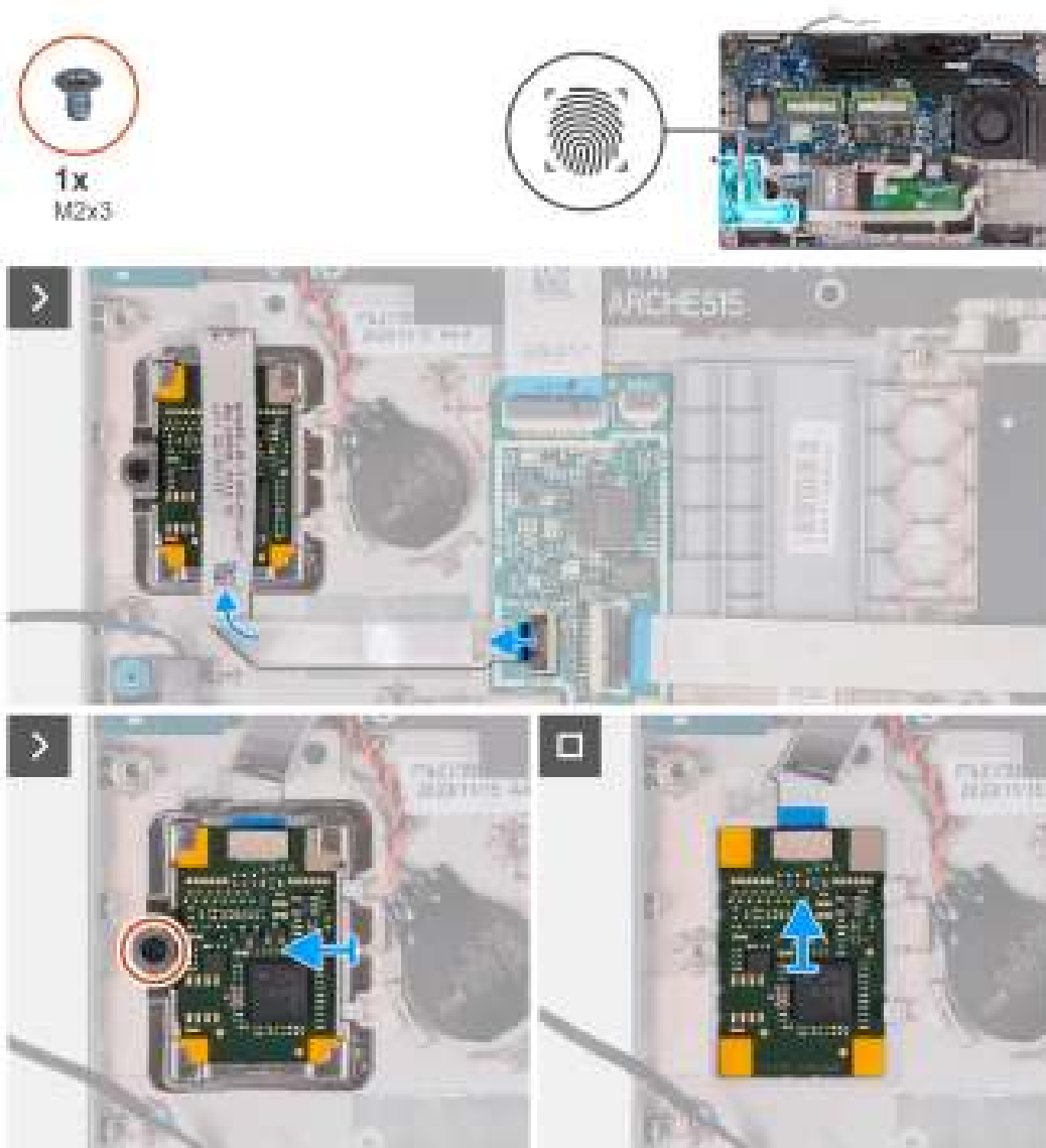
Afbeelding 94. De vingerafdrukkezer verwijderen
