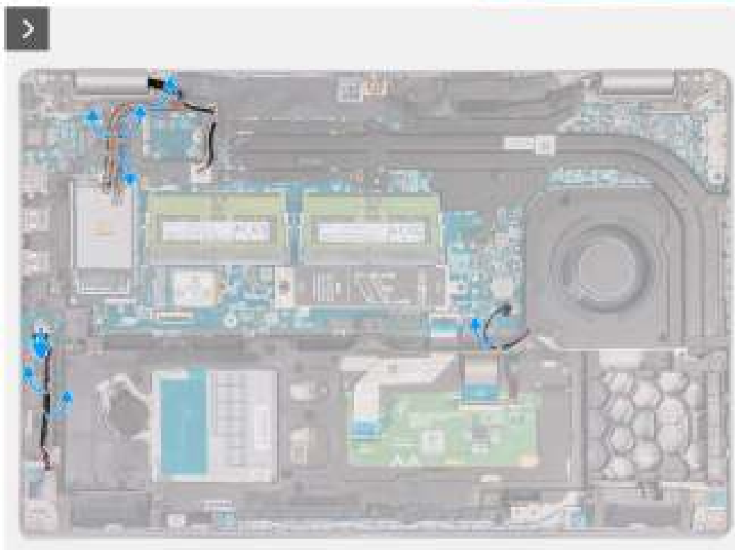
Afbeelding 37. Kabels verwijderen
