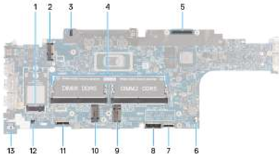
Afbeelding 52. Systeemkaartconnectoren
