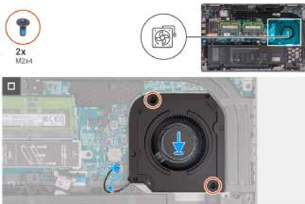
Afbeelding 34. De ventilator installeren
