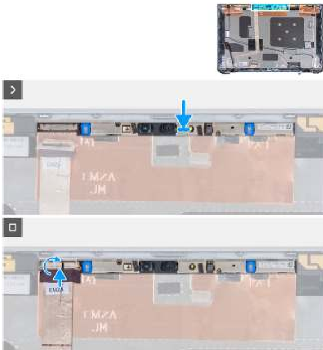
Afbeelding 85. De cameramodule installeren
