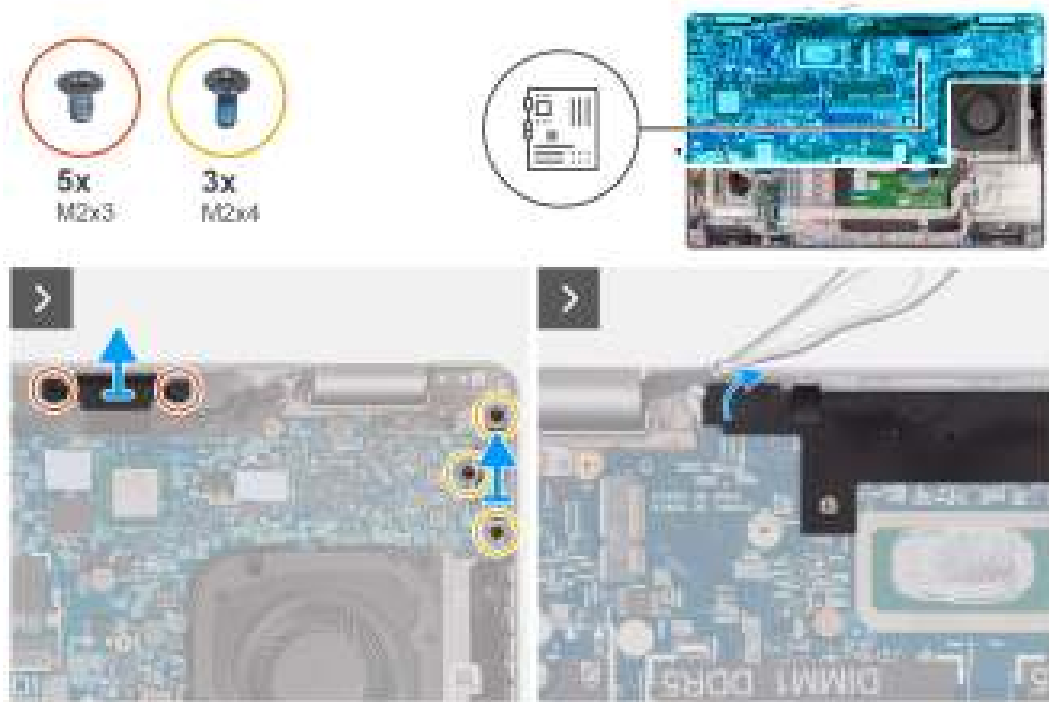
Afbeelding 53. De schroeven verwijderen
