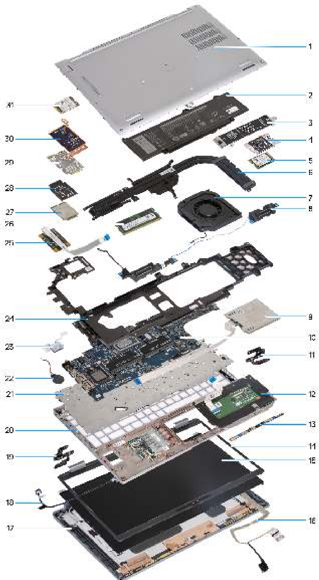
Afbeelding 10. Belangrijke componenten van uw computer
