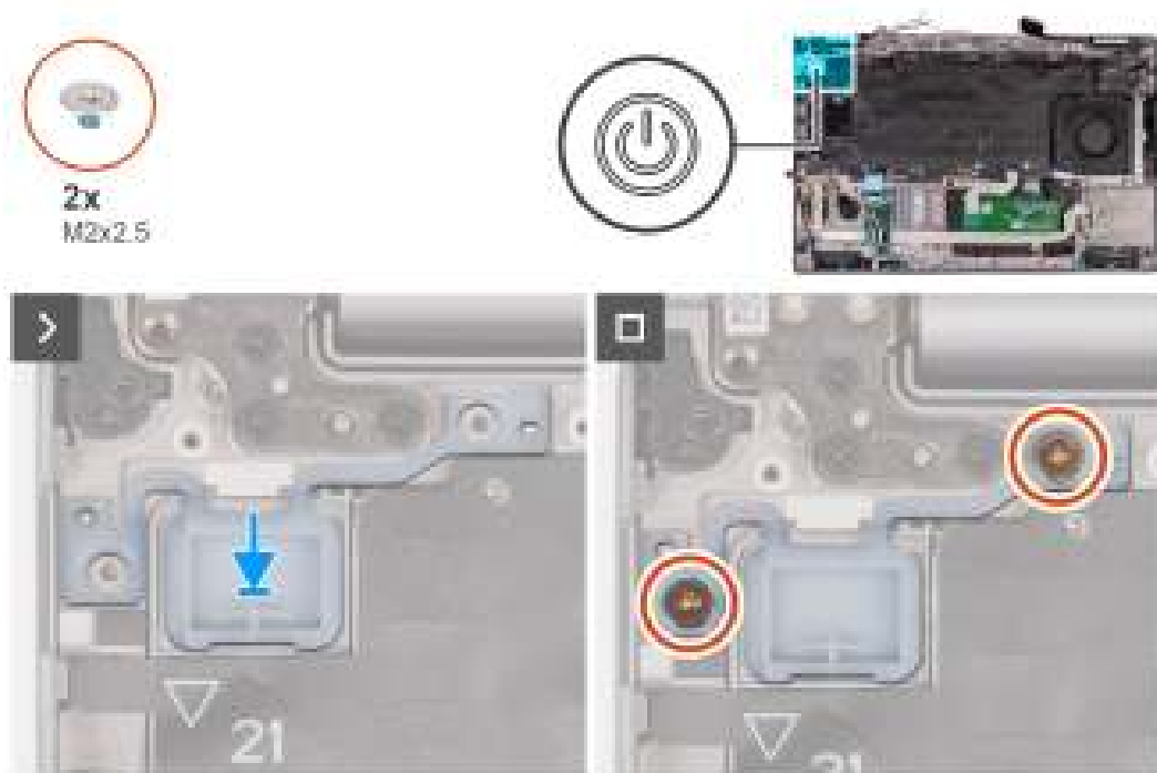
Afbeelding 62. De aan/uit-knop plaatsen
