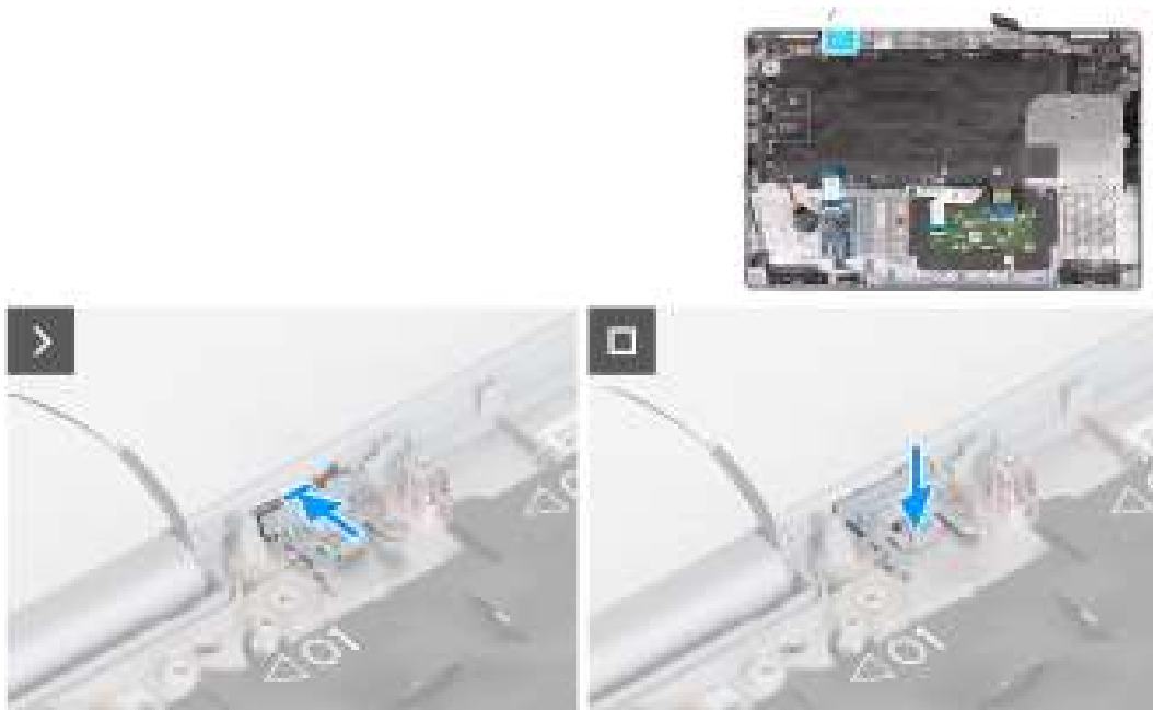
Afbeelding 99. De dummy simkaartslotvuller installeren
