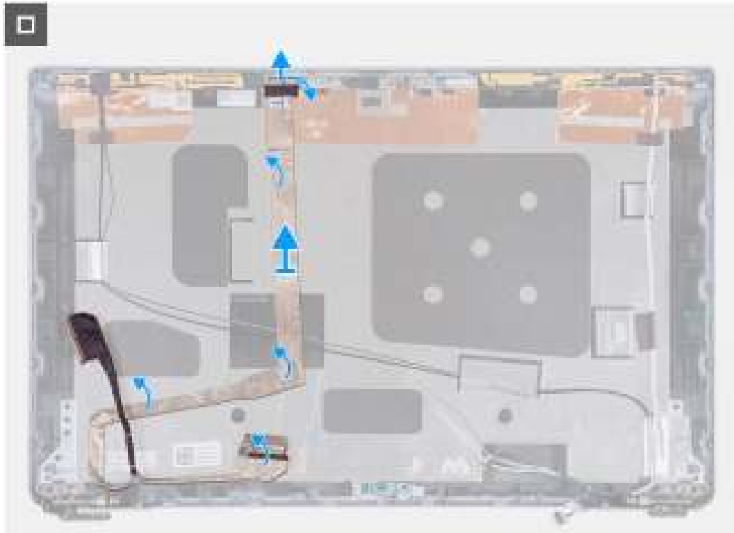
Afbeelding 90. De beeldschermkabel verwijderen
