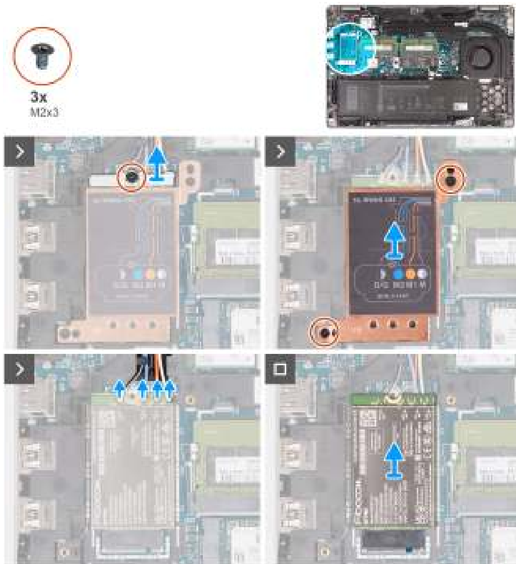
Afbeelding 23. De 5G WWAN-kaart verwijderen
