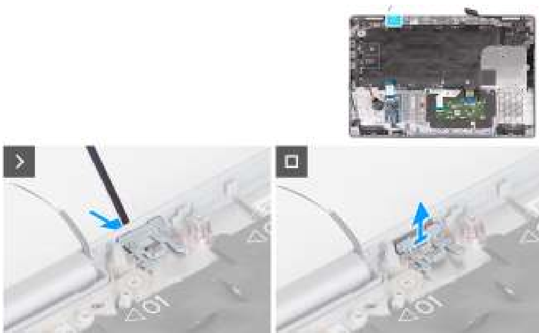
Afbeelding 98. De dummy simkaartslotvuller verwijderen
