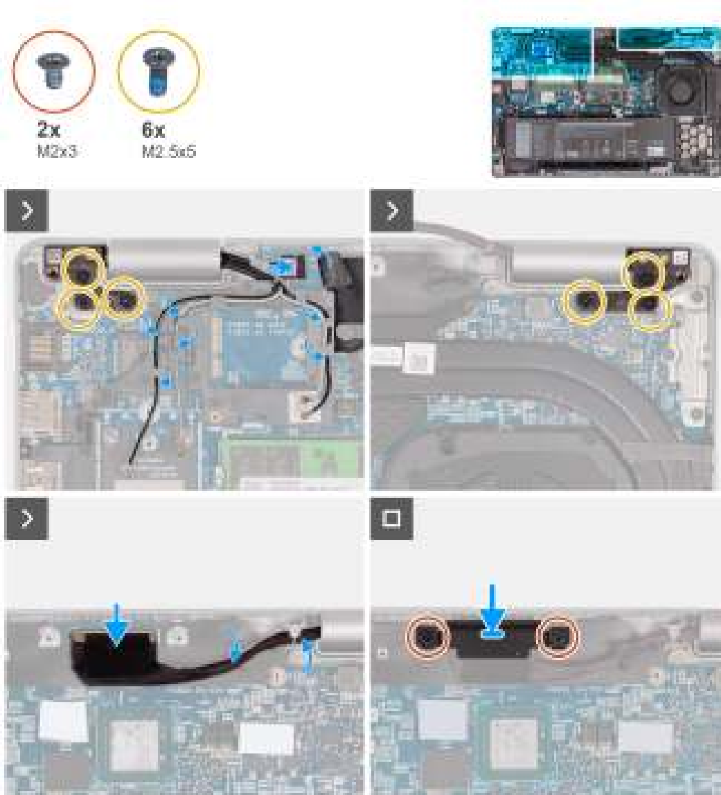
Afbeelding 73. De beeldschermeenheid plaatsen
