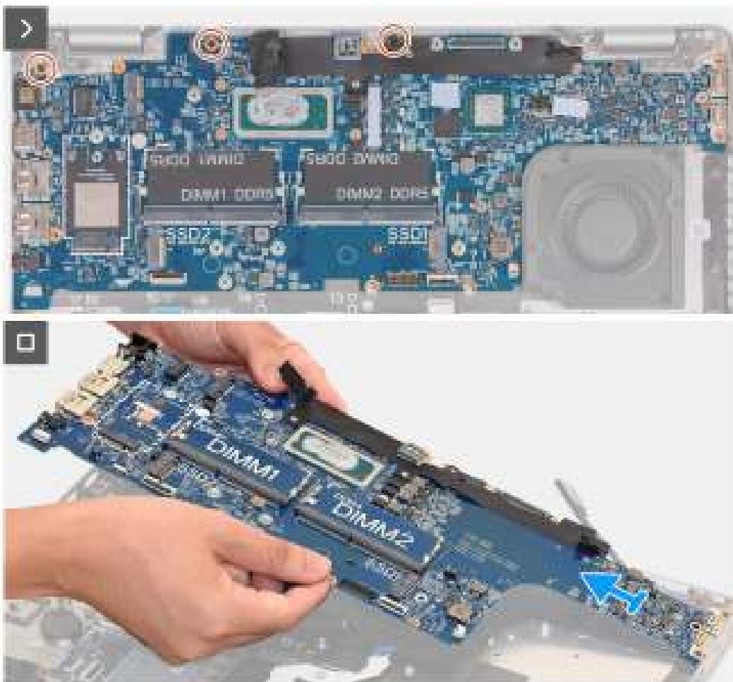
Afbeelding 55. De systeemkaart verwijderen
