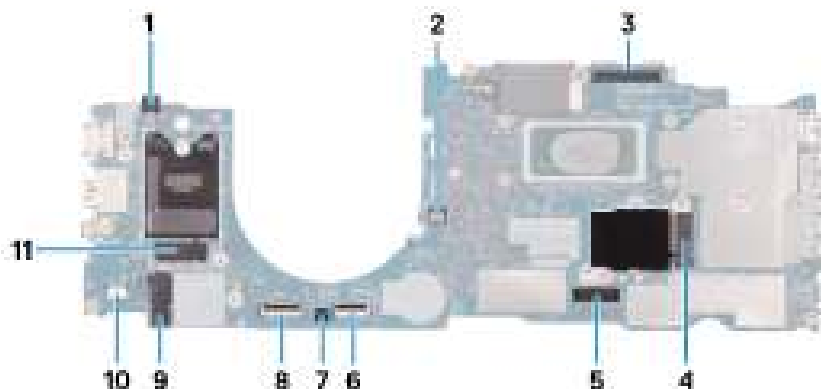
Afbeelding 48. Systeemkaartconnectoren
