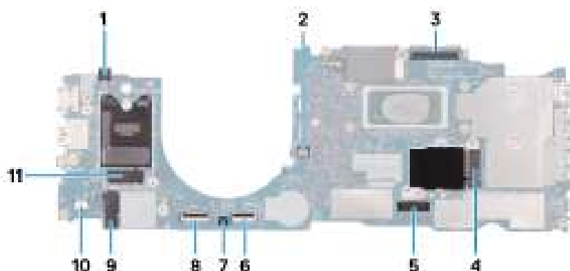
Afbeelding 44. Systeemkaartconnectoren
