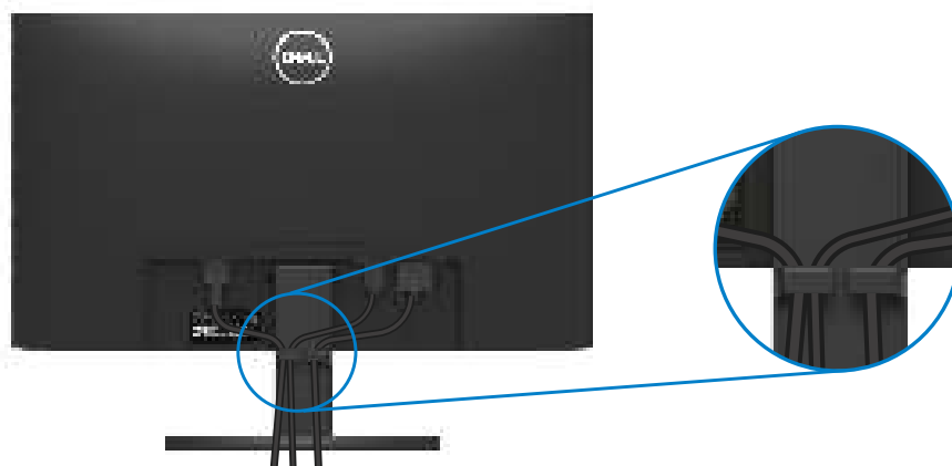
Afbeelding 19. Kabels ordenen
