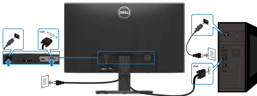
Afbeelding 17. VGA-kabel aansluiten
